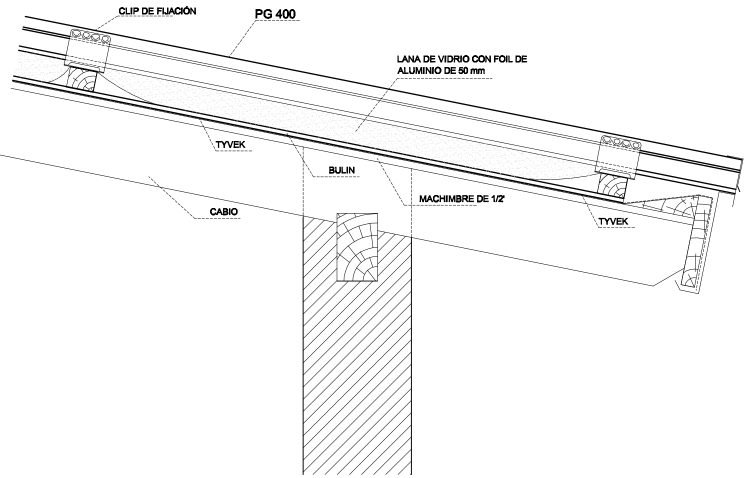
DETALLE CUBIERTA CON ESCURRIMIENTO LIBRE ESTRUCTURA DE MADERA
