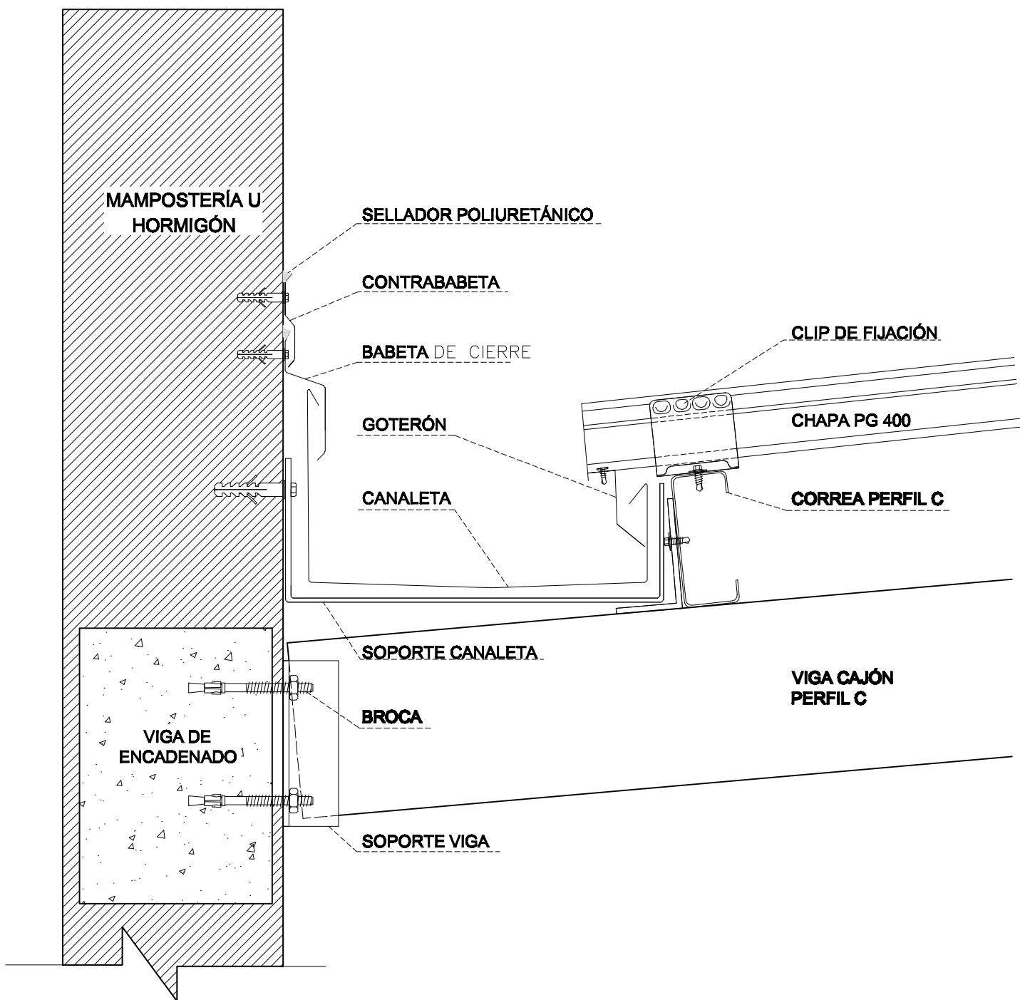
DETALLE CANALETA PG 400
